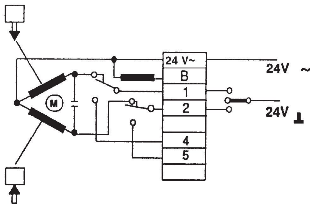
ML 6425B3005 (24 V, funkcja awaryjna)
