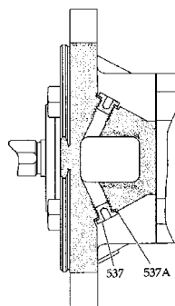
Przekrój E-E
