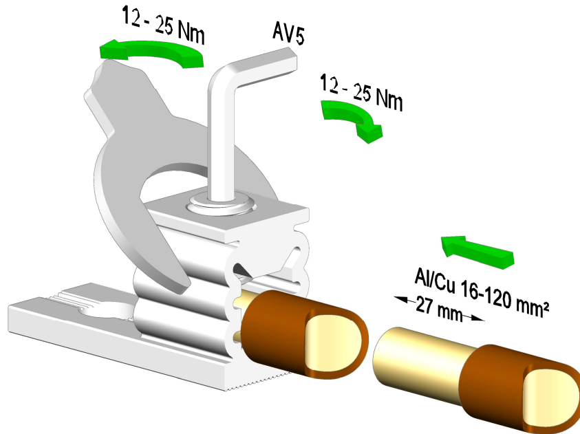
KIRISTYS- JA VASTAMOMENTTI TIGHTEN- AND REVERSE TORQUE
