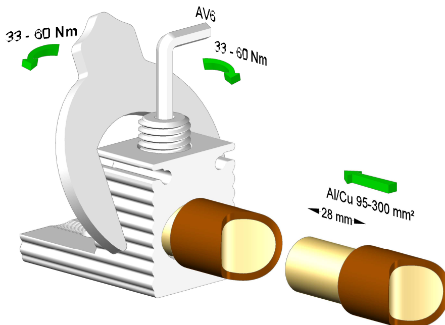
KIRISTYS- JA VASTAMOMENTTI TIGHTEN- AND REVERSE TORQUE
